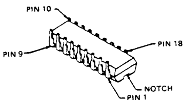
M54563P (Q1038) M54564P (Q1040)
