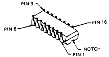
μPD4094BC (Q2001)
