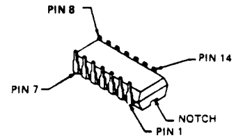
CX-7925B (Q2018,2024)
